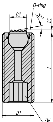
Forma F sfera in acciaio spianata, zigrinata
