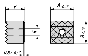
Forma A acciaio per utensili
