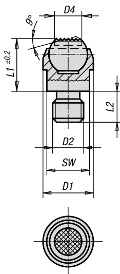
Forma M con gambo filettato, sfera spianata, con inserto zigrinato in metallo duro
