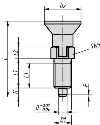
Forma C con incavo d'arresto, senza controado
