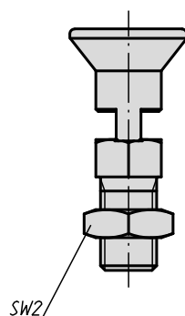
Forma D con incavo d'arresto, con controado
