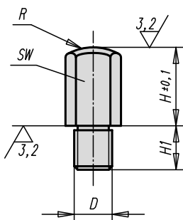
Forma C superficie convessa temprata
