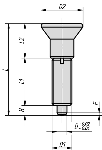
Perno di arresto con rondella di avvitamento
