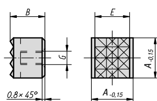
Forma B zigrinatura in metallo duro
