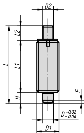
Forma J con perno filettato senza controdamo
