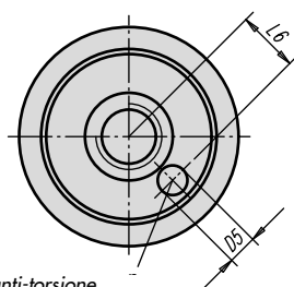
Foro per la spina anti-torsione
