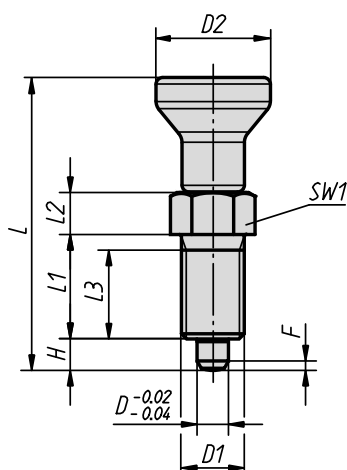
Forma C con incavo d'arresto, senza contro dado
