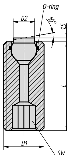
Forma K sfera in Delrin, spianata, liscia
