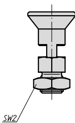
Forma D con incavo d'arresto, con controdamo
