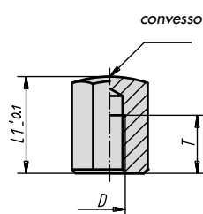
Forma E foro filettato e superficie convessa
