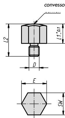
Forma B gambo filettato e superficie convessa
