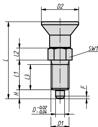
Forma A senza incavo d'arresto, senza controado
