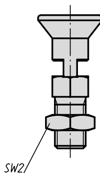
Forma D con incavo d'arresto, con contro dado
