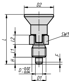
Forma C con incavo d'arresto, senza controdamo
