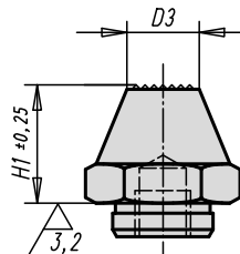
Forma C appoggio zigrinato
