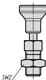
Forma B senza incavo d'arresto, con contro dado
