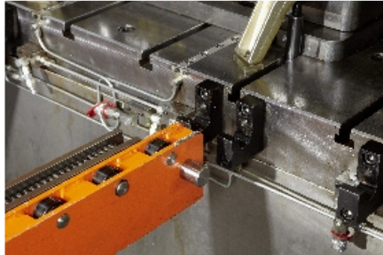
La consolle viene accostata alla pressa...
